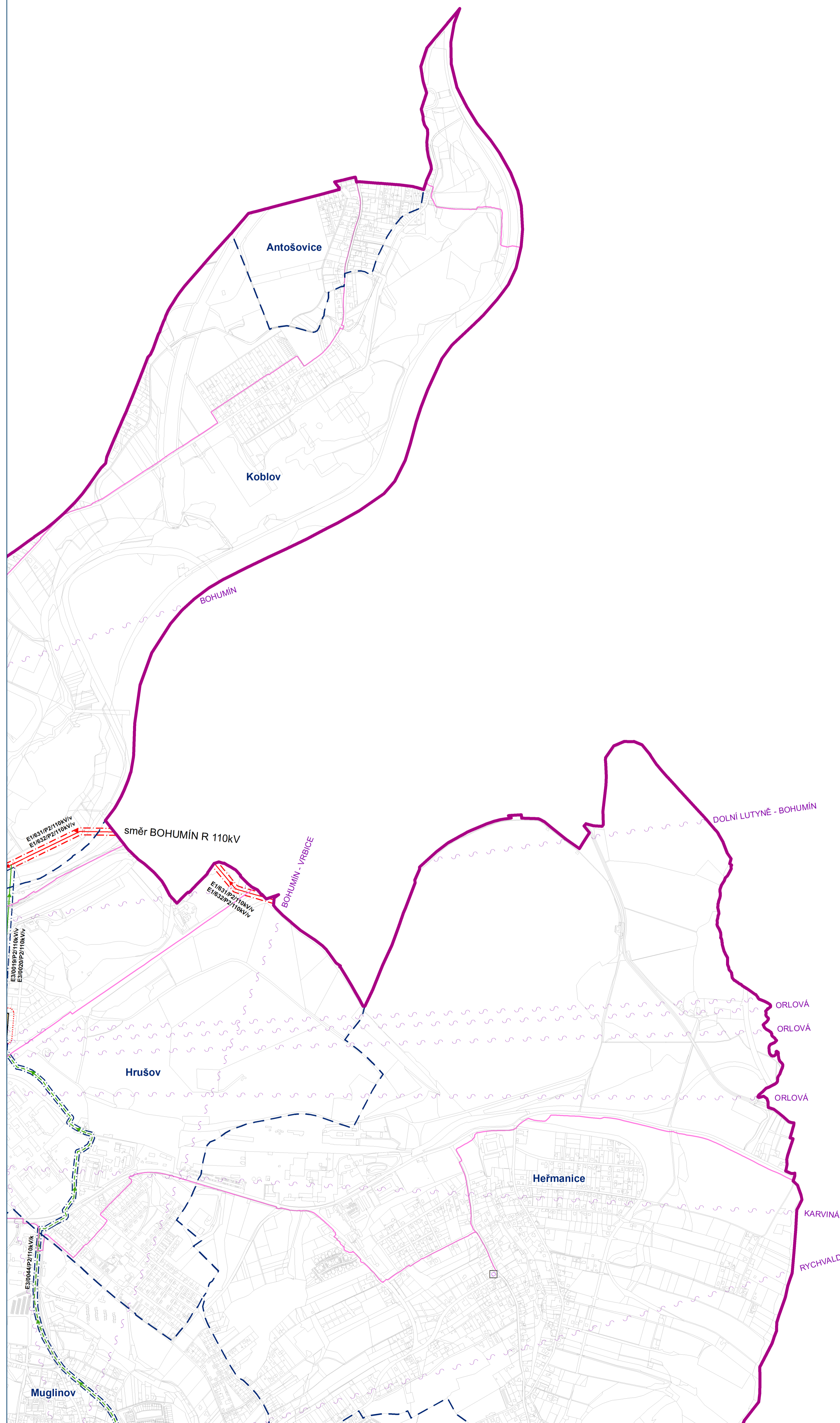
HLAVNÍ VÝKRES Koncept veřejné infrastruktury - zásobování elektřinou a telekomunikace
