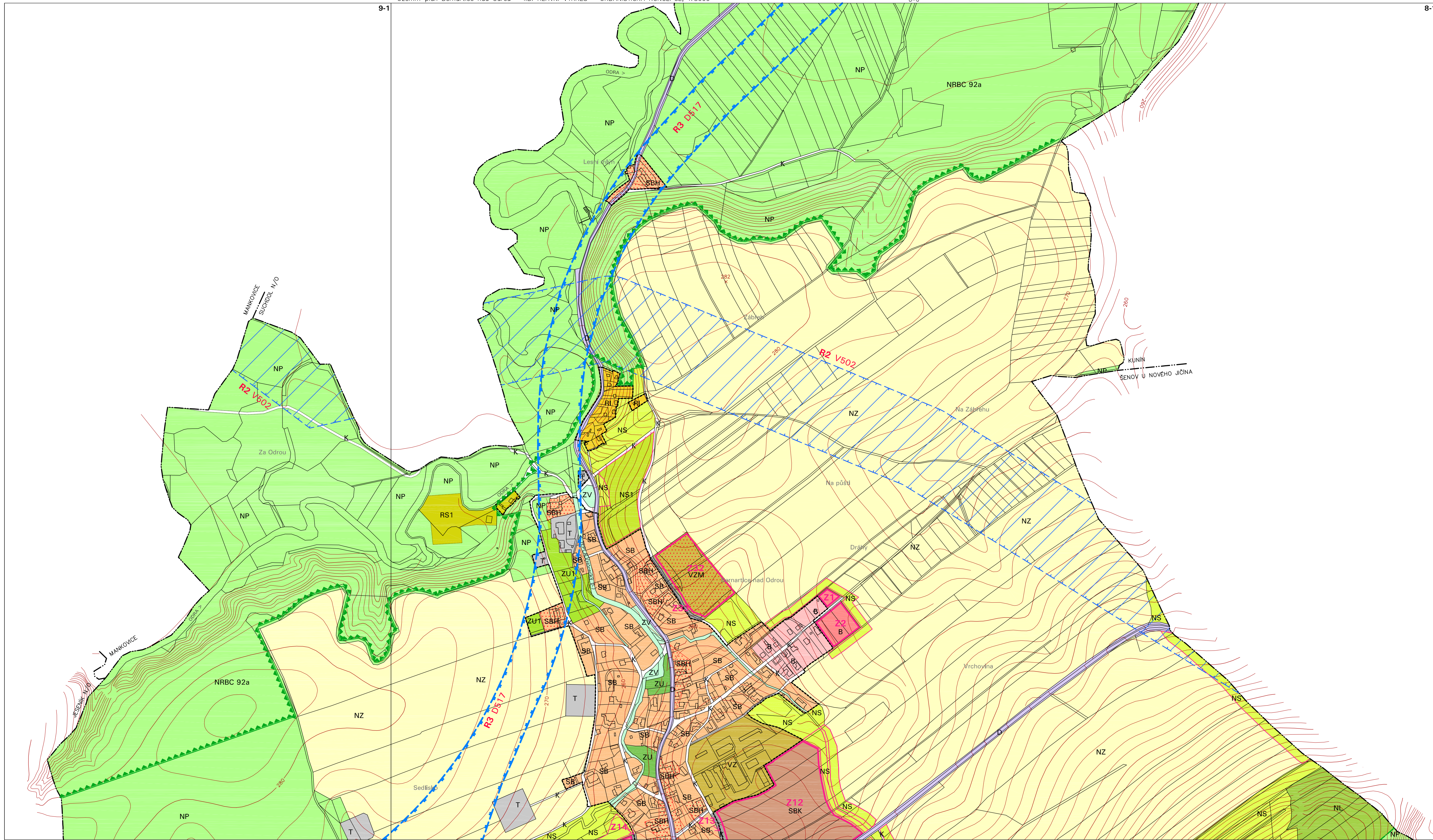
Územní plán Bernartice nad Odrou – I.B. HLAVNÍ VÝKRES – URBANISTICKÁ KONCEPCE, 1:5000
