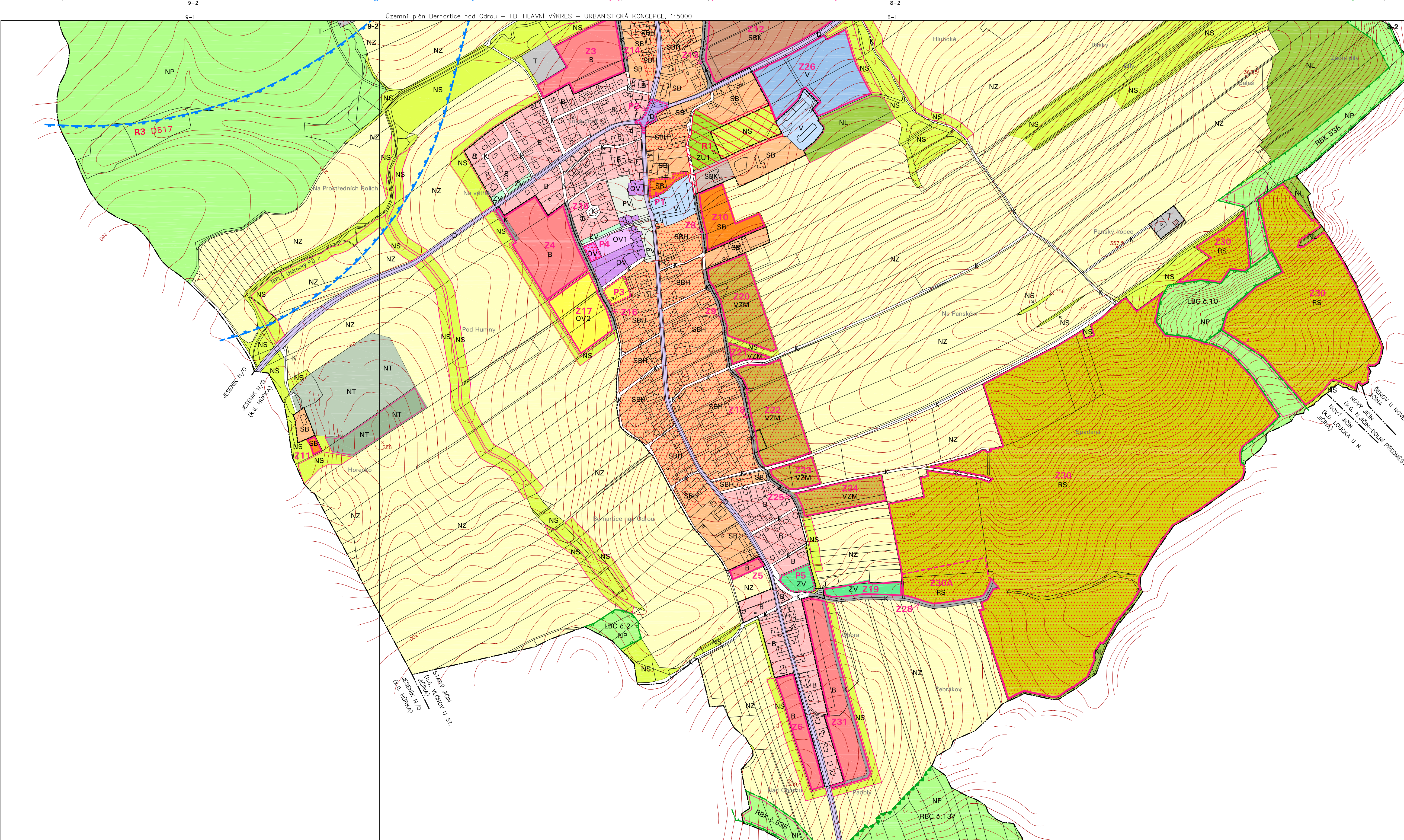
Územní plán Bernartice nad Odrou – I.B. HLAVNÍ VÝKRES – URBANISTICKÁ KONCEPCE, 1:5000
